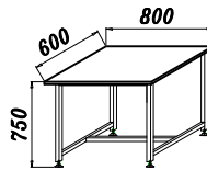
独立工作台
